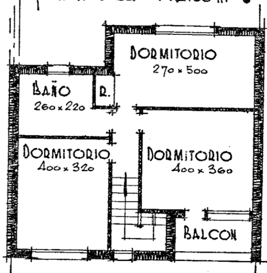
PLANTA ALTA
