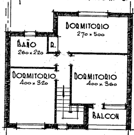
PLANTA ALTA
