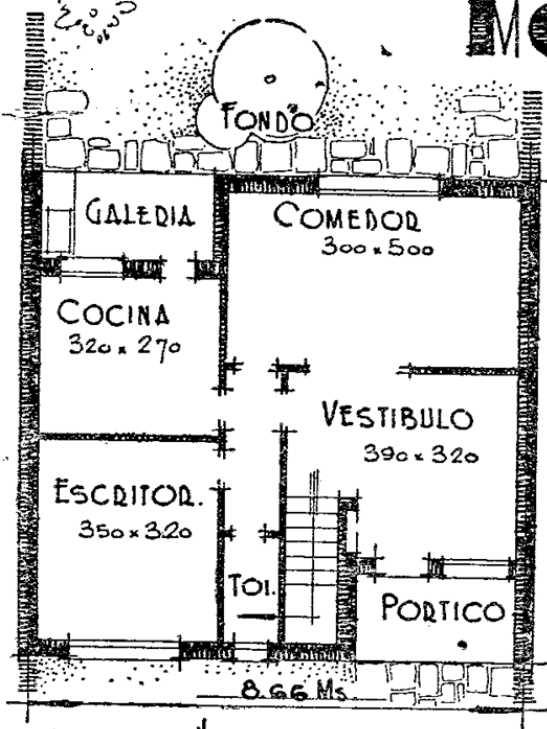
PLANTA BAJA
