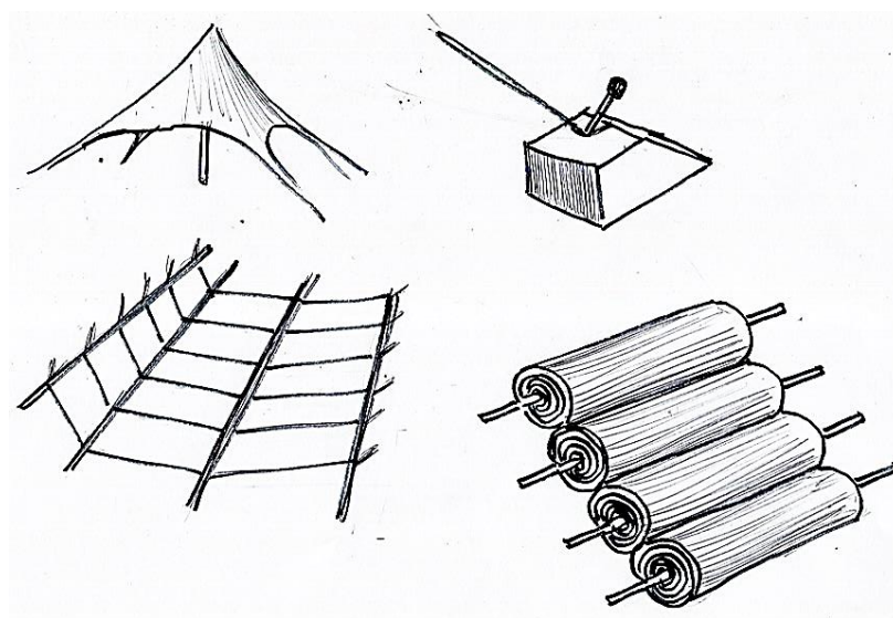
OTRA PROPUESTA DE LA CUBIERTA TENSADA
